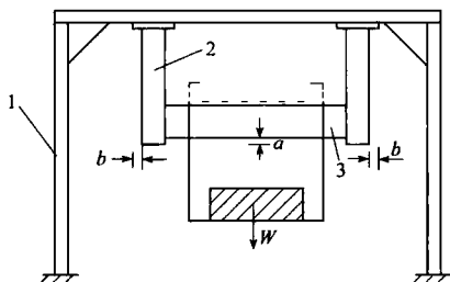
图 B.0.3-3 吊架固定体和定位方式
