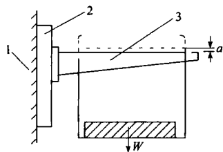
图 B.0.3-1 支架固定体和定位方式
