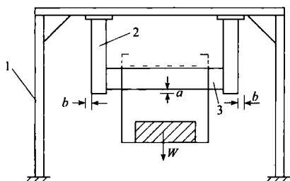
图 B.0.3-2 支架固定体和定位方式
