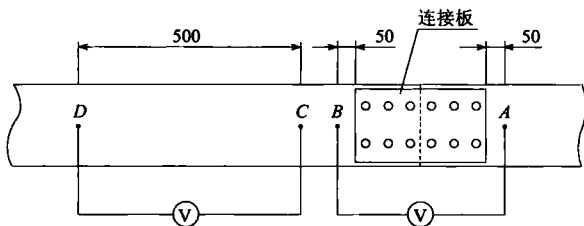
图 C.0.2 电气连续性试验布置
